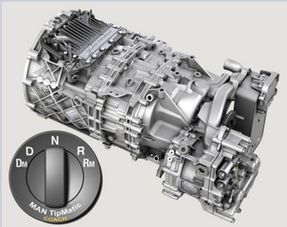
MAN TipMatic® Coach - 12-stopenjski avtomatski menjalnik z Easy-Start (ZF 12 AS)
