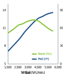
1,2-LITRSKI BENCINSKI MOTOR MPI
