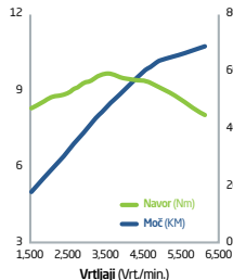
1,0-LITRSKI BENCINSKI MOTOR MPI
