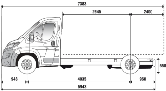
L3 - ŠASIJA S KABINO
