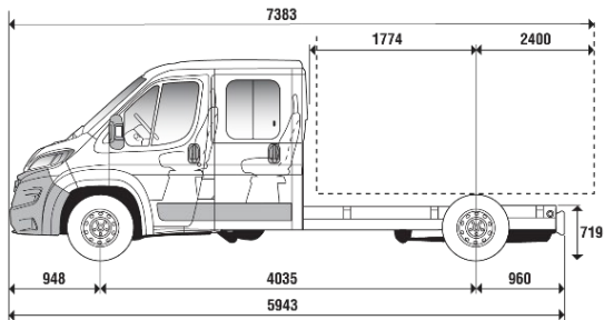
L3 - ŠASIJA Z DVOJNO KABINO
