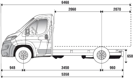
L2 - ŠASIJA S KABINO
