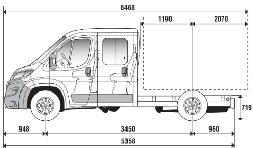
L2 - ŠASIJA Z DVOJNO KABINO
