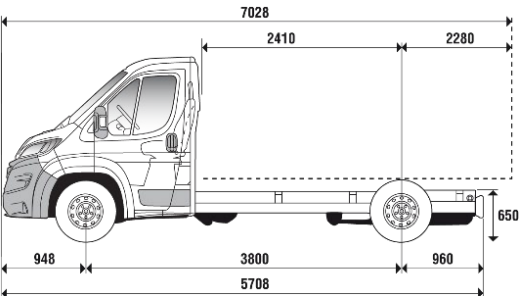
L2+ - ŠASIJA S KABINO
