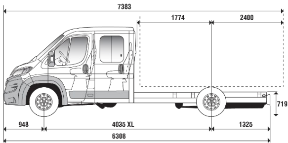
L4 - ŠASIJA Z DVOJNO KABINO
