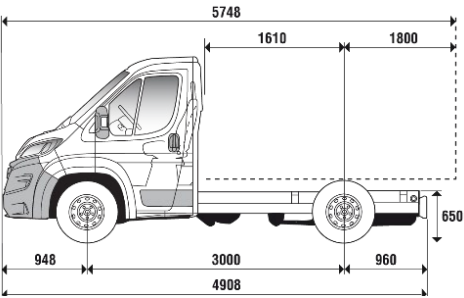
L1 - ŠASIJA S KABINO
