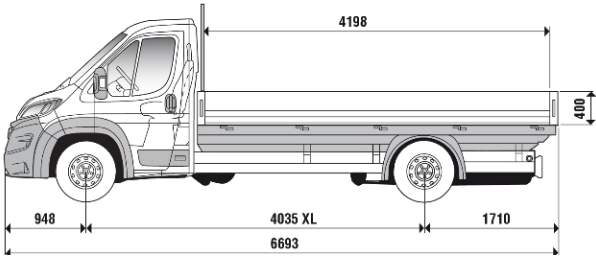
L4 - ŠASIJA S KABINO IN TOVORNI KESON
