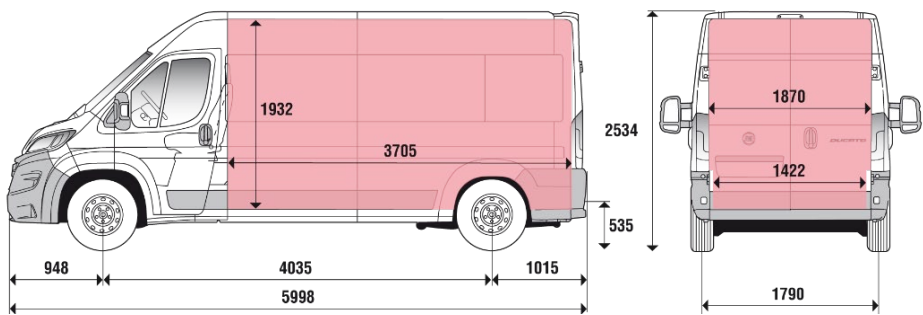
FURGON - L3H3 - 15 M 3
