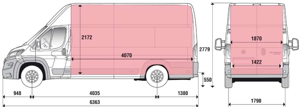
FURGON - L4H3 - 17 M 3
