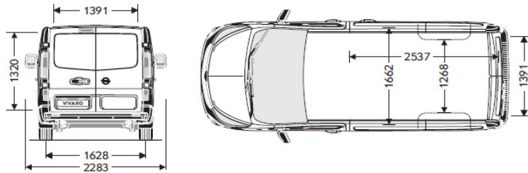
Vivaro Van L2H2
