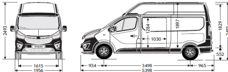
Vivaro Van L2H2
