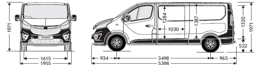
Vivaro Van L2H1
