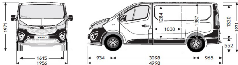
Vivaro Van L1H1
