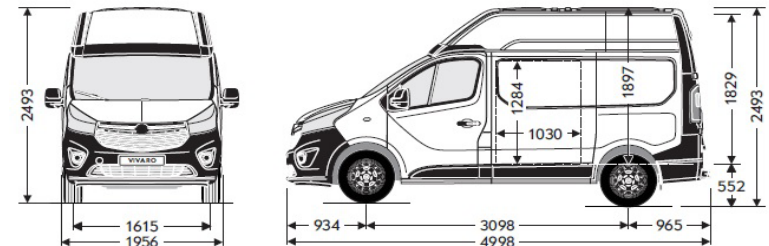
Vivaro Van L1H2
