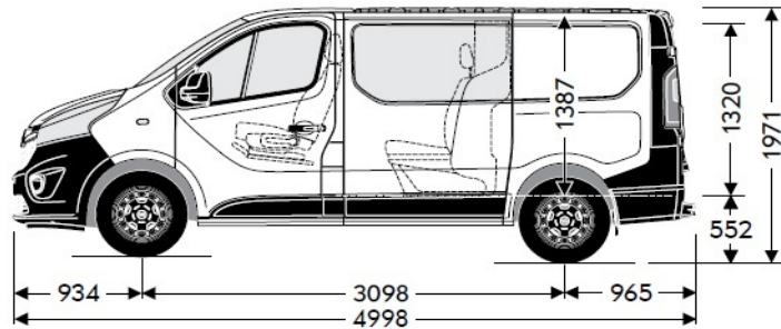
Vivaro Crew Van L1H1
