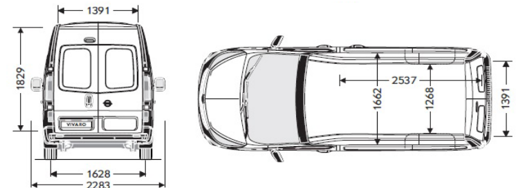
Vivaro Van L2H1
