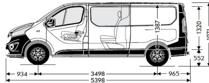
Vivaro Crew Van L2H1
